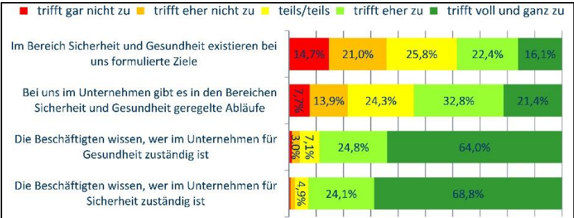
Abbildung 13: Strukturen (Multiplikatoren)
