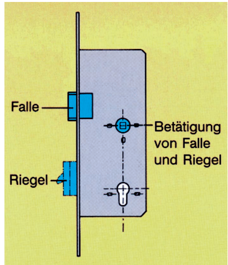
Bild 2: Panikschloss
